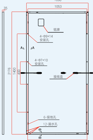
后视图
