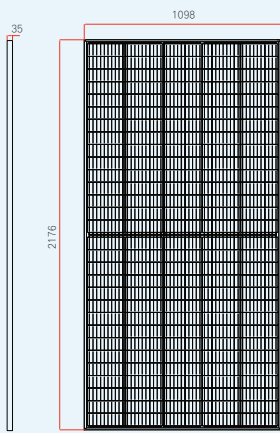
正视图
