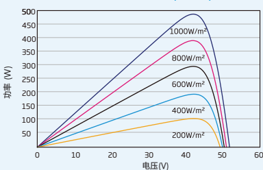
组件的P-V曲线 (490W)
